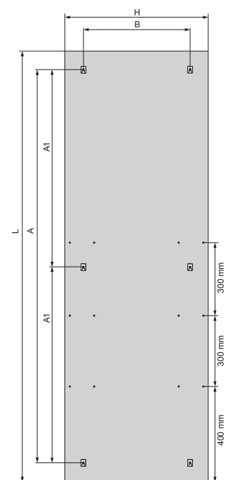
Calentadores con 1.800 mm de altura
