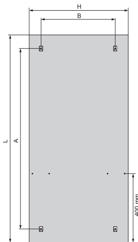
Calentadores con 1.200 mm de altura
